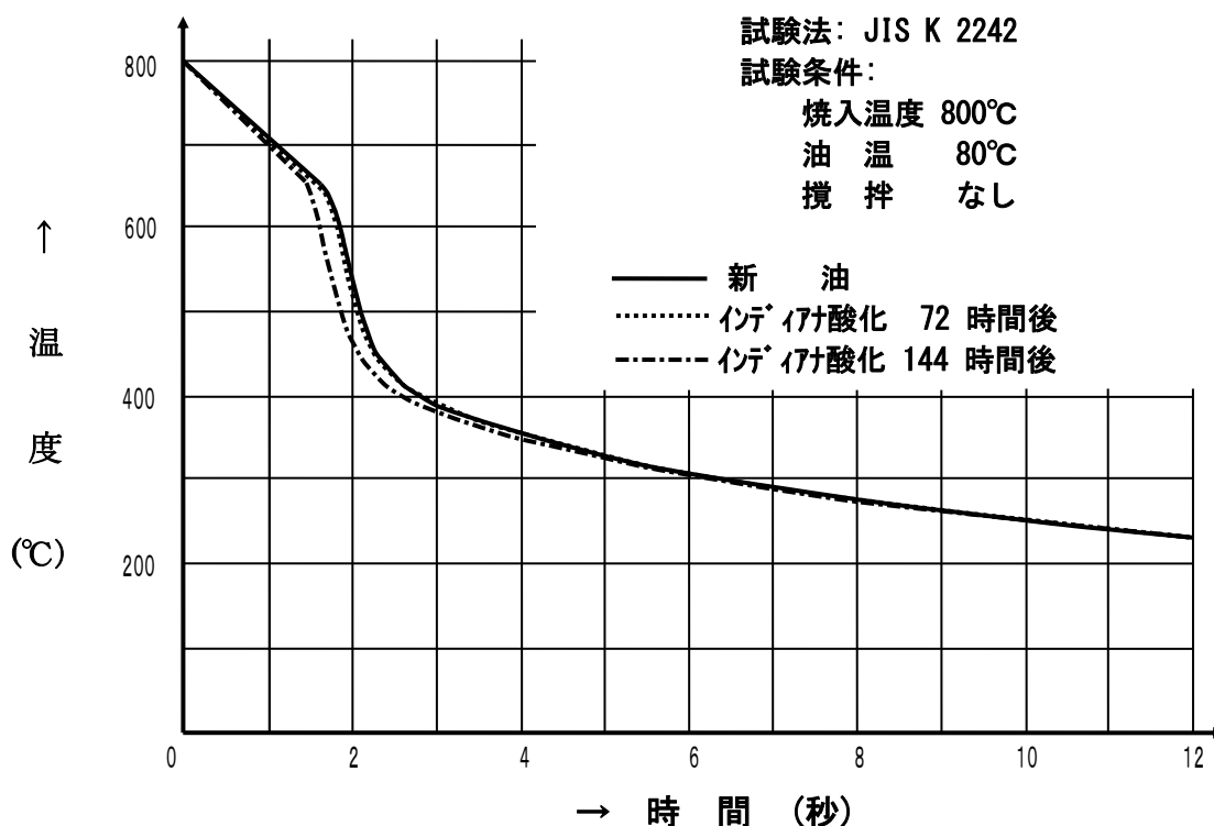
焼 入 油 冷 却 曲 線 例
