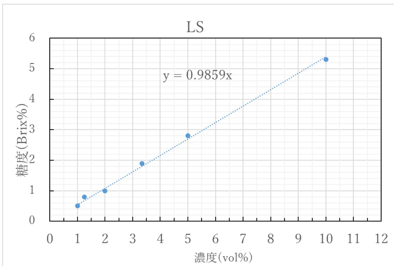
糖度－濃度線図
